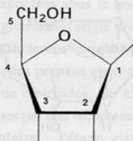
\beta -D-ribofuranose
