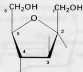
\alpha -D-fructofuranose
