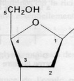
\beta -D-2-désoxy-ribofuranose
