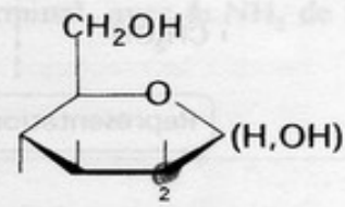
D-mannopyranose épimère en C2
