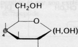
D-galactopyranose épimère en C4
